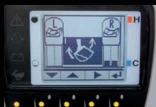
Réglage du débit d'huile maxi (aux. 1 et aux. 2)
